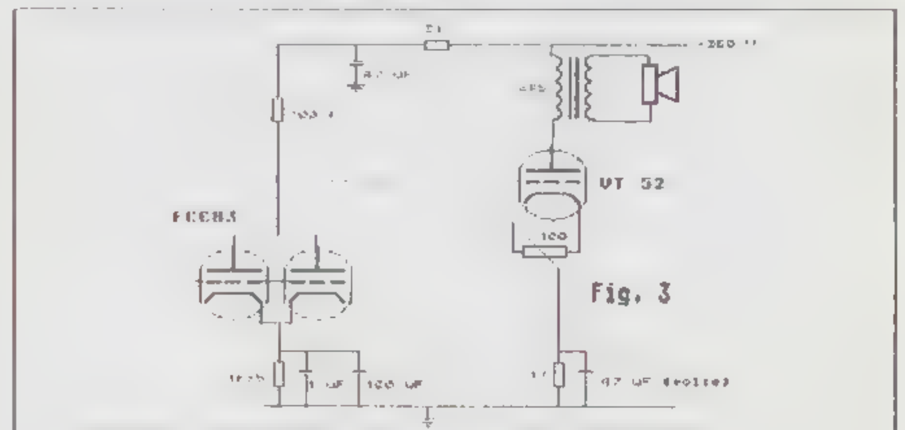
De schakeling van l'Audiophile uit 1988
